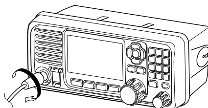
Connecteur du microphone
