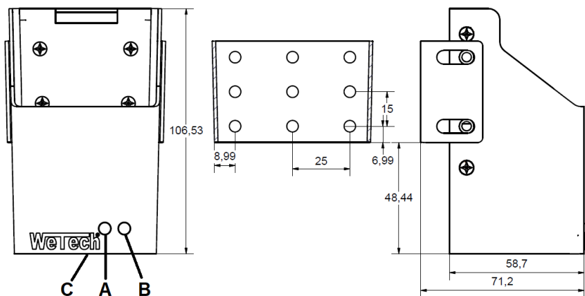
Schemazeichnung WTC642
