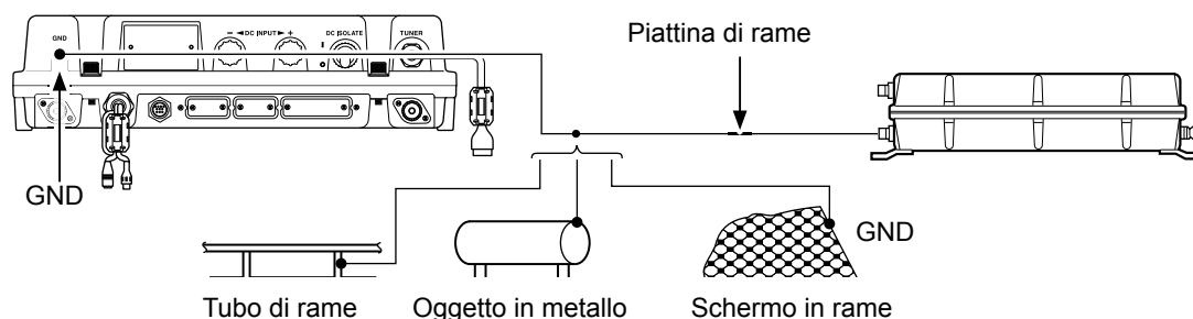
Esempio di impianto di terra
